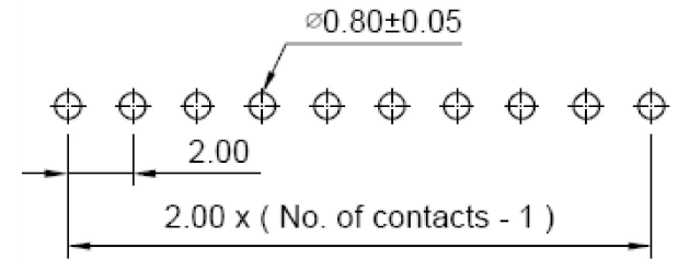
P.C.Board Layout
